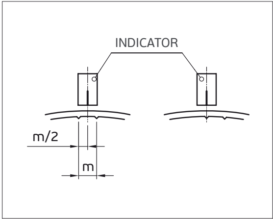
Fig. n.º16. Wear indicator
